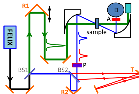
FIG. 2. The apparatus.
