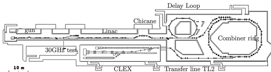
FIG. 4. CTF3 layout.
