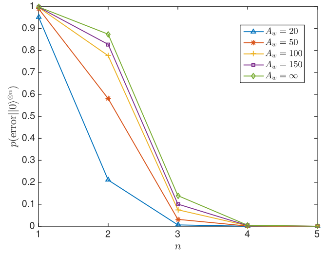
(a) q_{1 \rightarrow 0} = q_{0 \rightarrow 1} = 0.05
