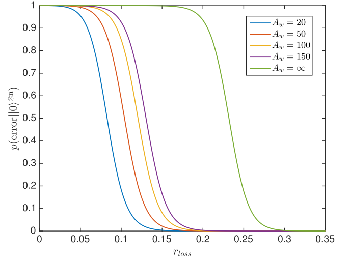
(a) q_{1 \rightarrow 0} = q_{0 \rightarrow 1} = 0.05
