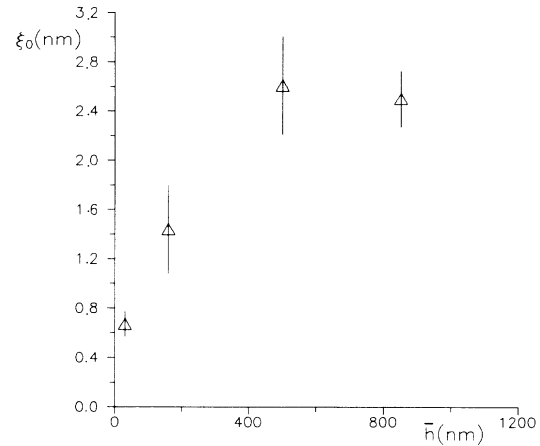
FIG. 7. \xi_0 vs \bar{h} plot.
