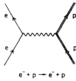
e^- + p \rightarrow e^- + p
