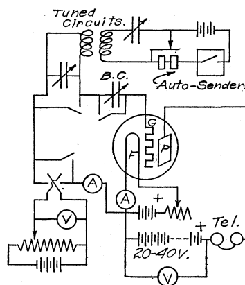
Fig. 2. Test circuit.
